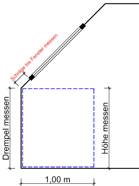
Beispiel-Schnitt Dachschräge
