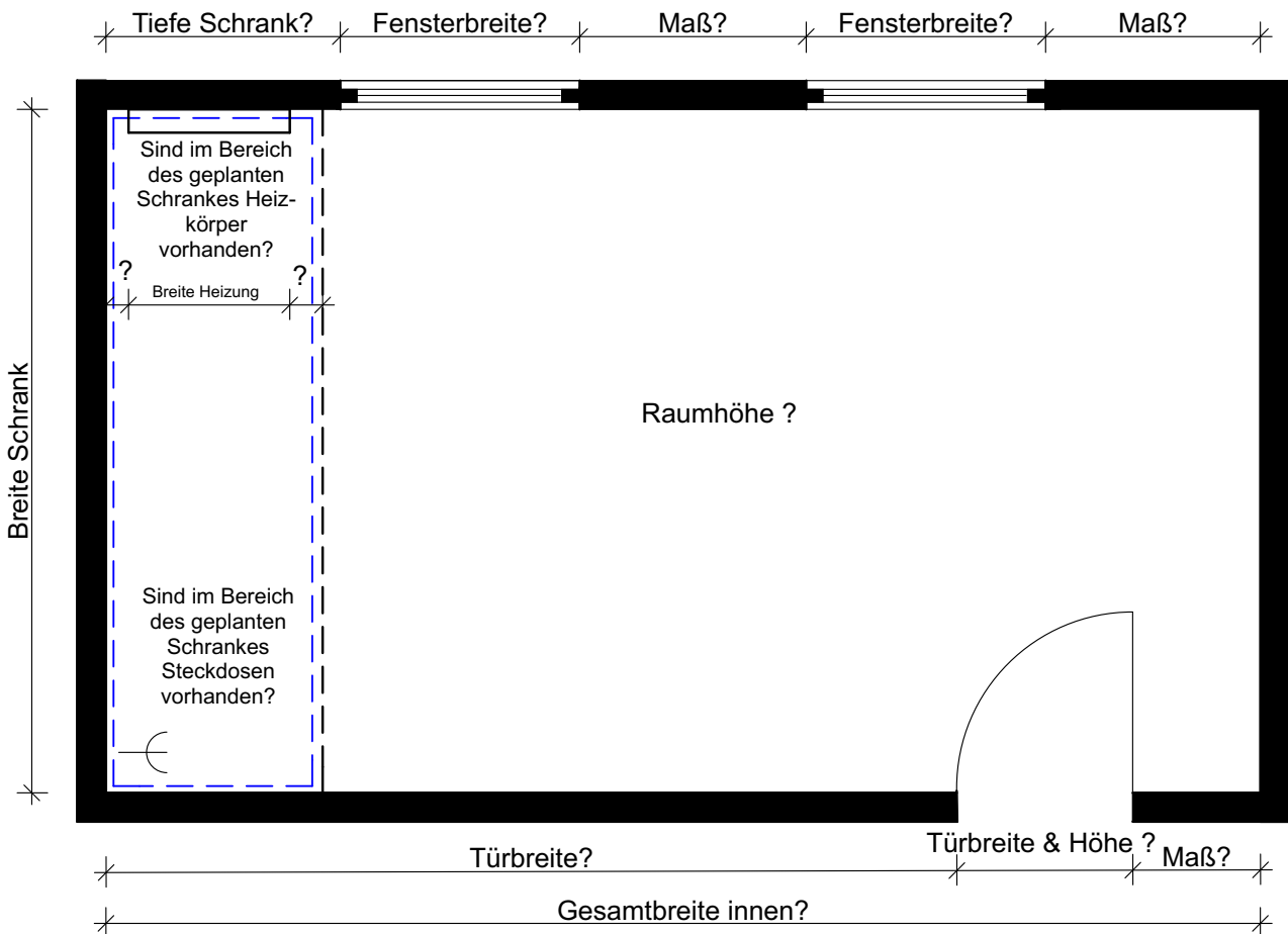
Beispiel-Grundriss Dachschräge
